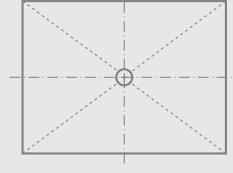
Fundo Primo, zemin elemanı dikdörtgen, merkezi olmayan gider, gider pozisyonu 1200 x 900 mm
